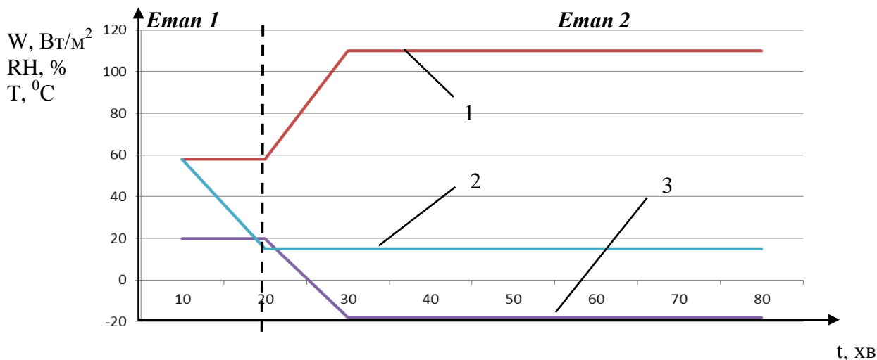
Рис. 1. Протокол порівняльних тестувань: 1 – енерговитрати суб’єкту W, Вт/м 2 ; 2 – відносна вологість навколишнього середовища RH, %; 3 – температура навколишнього середовища T, °C
